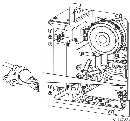
Prise pour réchauffeur de bloc-moteur
